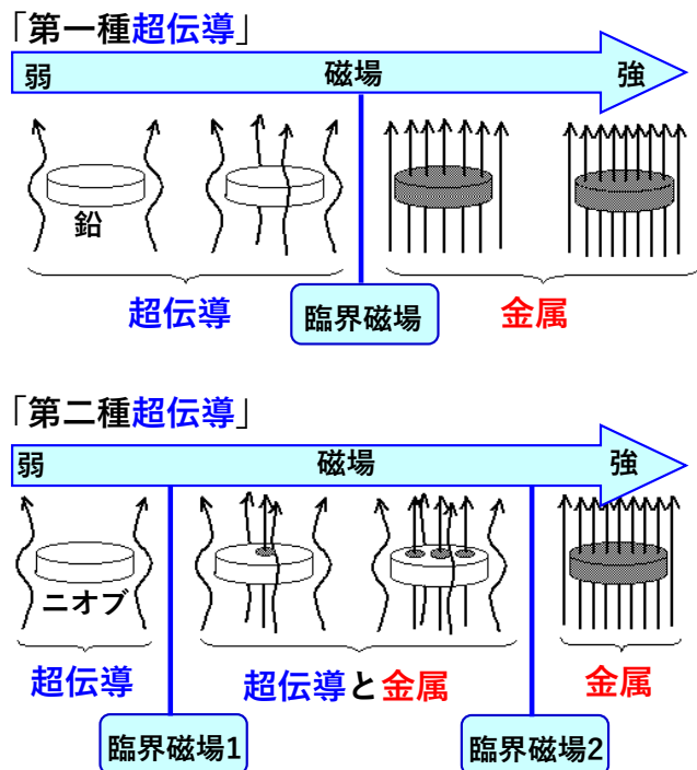
図2: 第一種超伝導と第二種超伝導。
